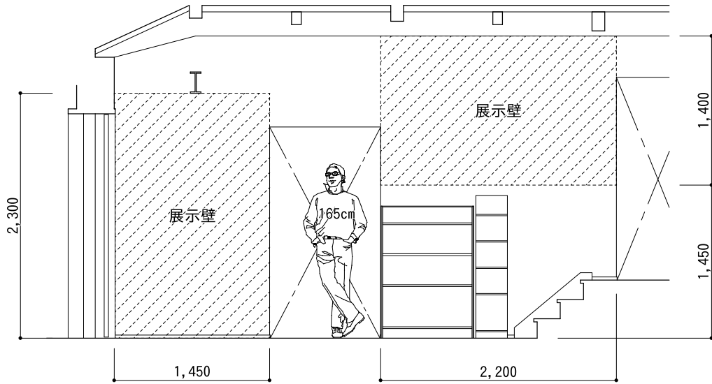
展開図 S=1/50
